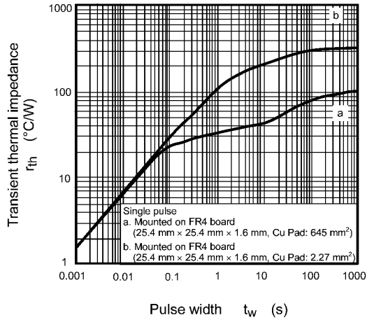
Fig. 8.13 r_{th} - t_w
